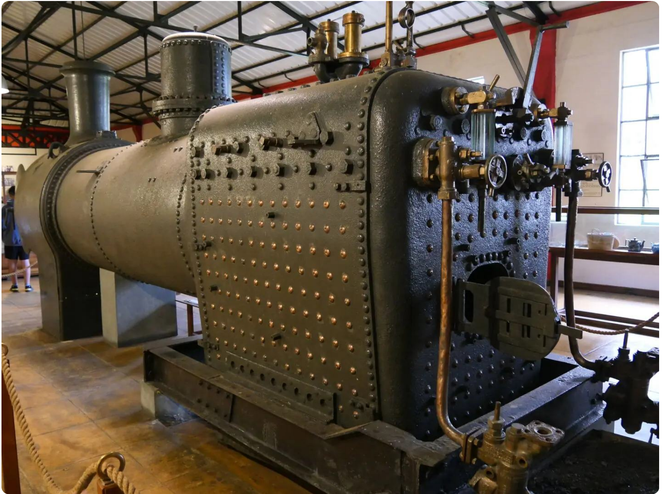
Autre ancienne machine de la fabrique de thé de Bois Chéri
